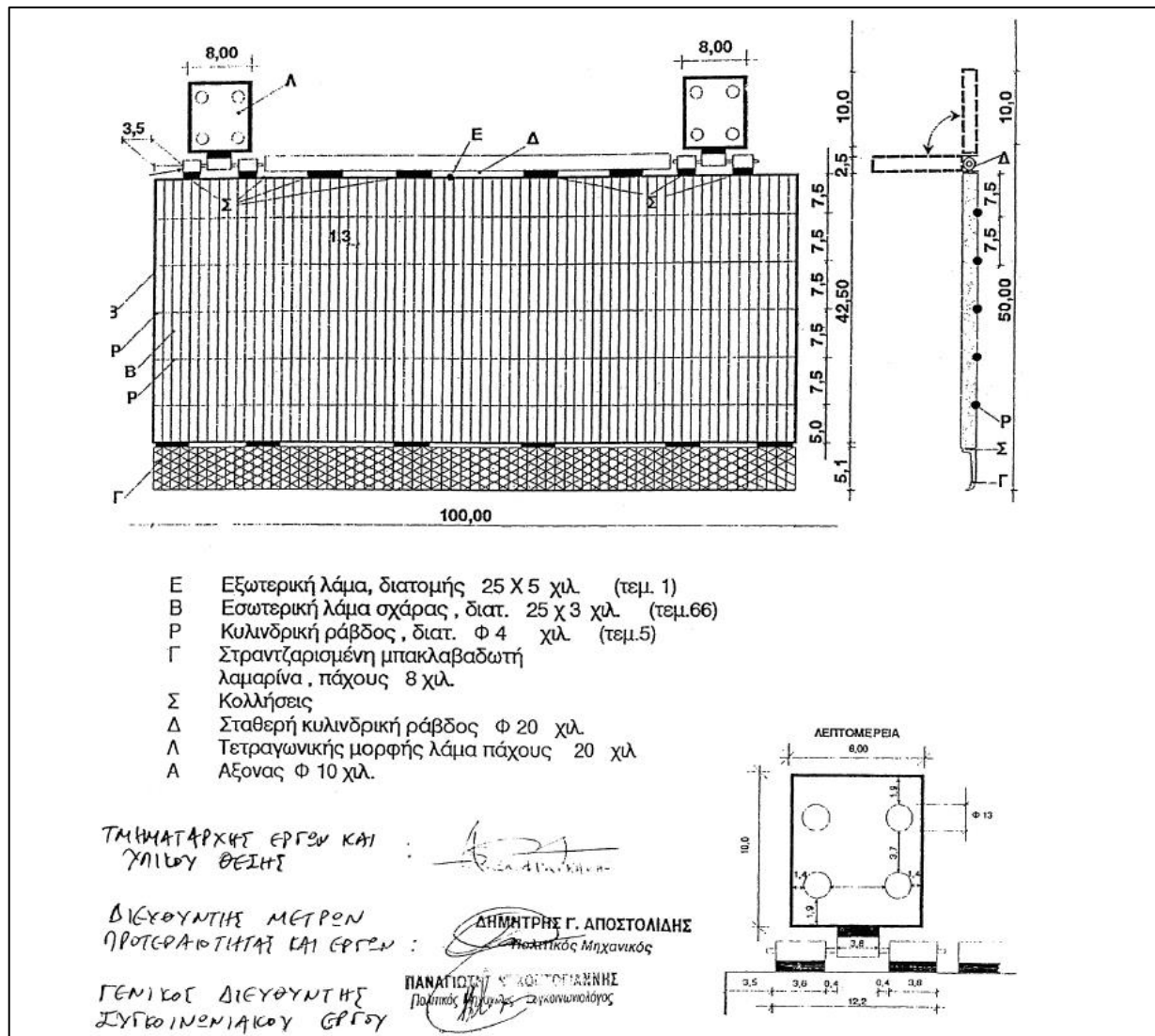
Εικόνα 1: Σχέδιο Κάτοψης Μεταλλικής Εσχάρας Σύνδεσης της Προεχού με το Πεζοδρόμιο
