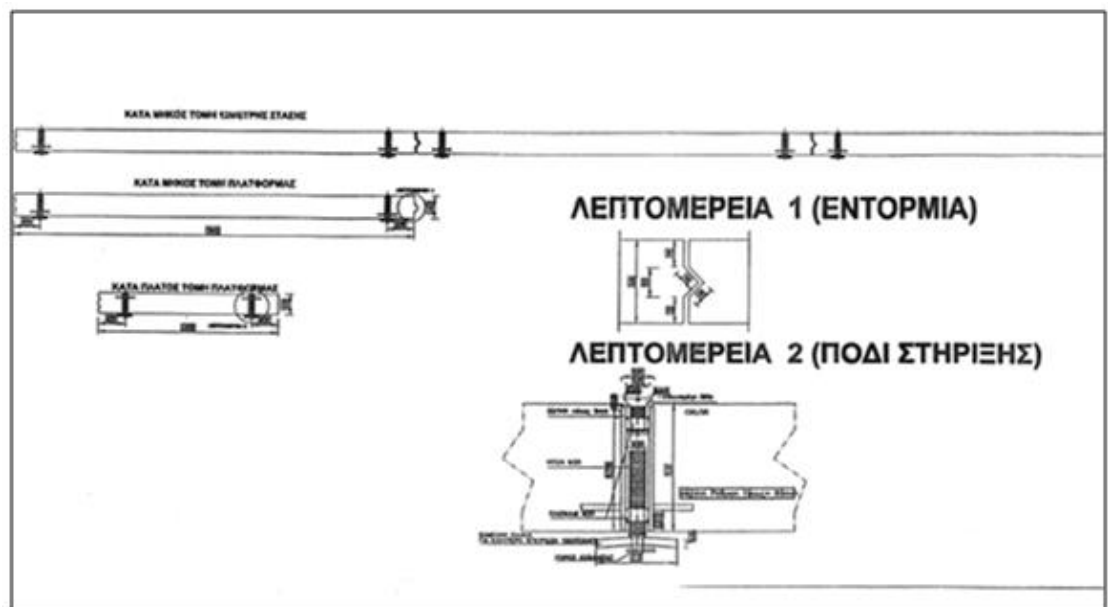
Εικόνα 3: Σχέδιο Τομής κατά πλάτος
